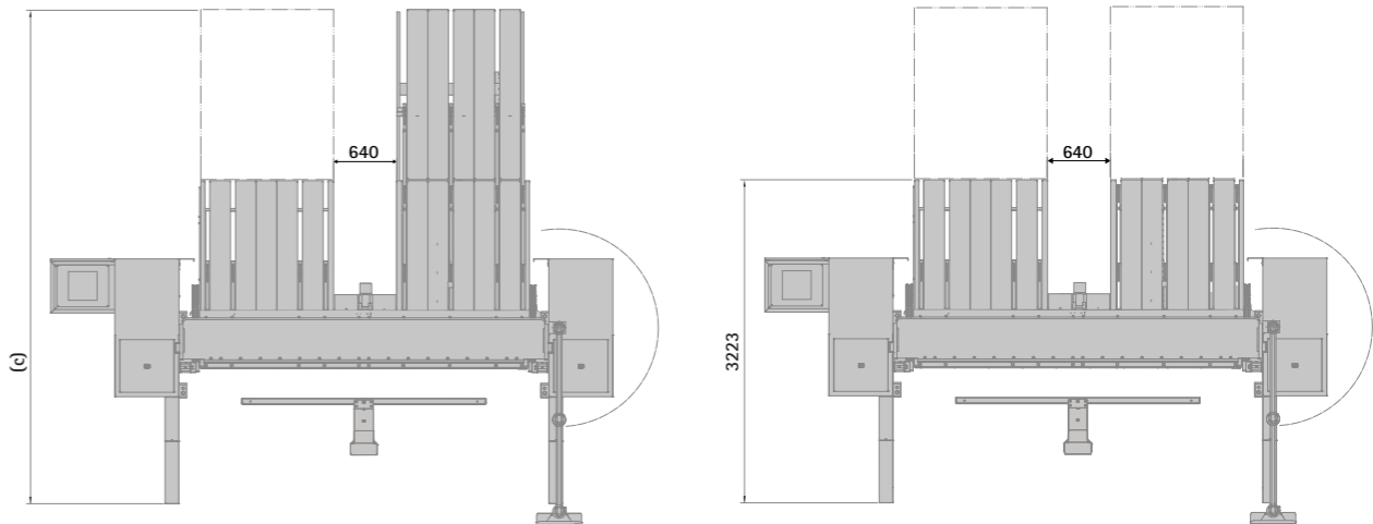
J-Form 3 200/1 600, 4 x 800 mm J-Form 4 000/1 600, 5 x 800 mm
