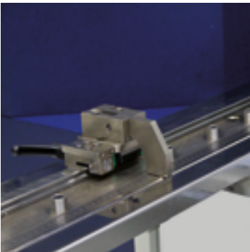
Winkelanschlag 1000 mm mit Maßstab inkl. seitlichem Klappanschlag auf Linearführung.
