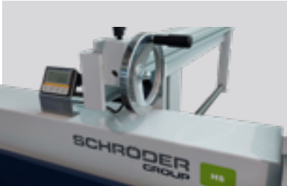
Optional: Manueller Hinteranschlag 750 mm von vorne verstellbar mit Digitalanzeige.
