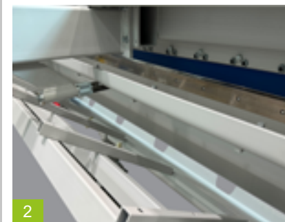
2 Blechochhaltevorrichtung nach vorne in abgekippter Stellung, pneumatisch gesteuert, incl. Blechrutsche, Anschlagtiefe 750 mm oder 1000 mm
