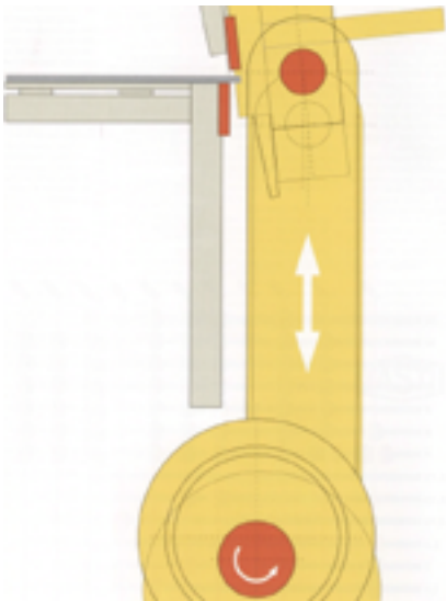
Kulissen geführter Messerbalken mit Exzenter angetrieben.
