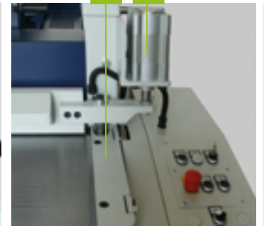
[3] Justierbarer Winkelanschlag [4] Pneumatischer Niederhalter
