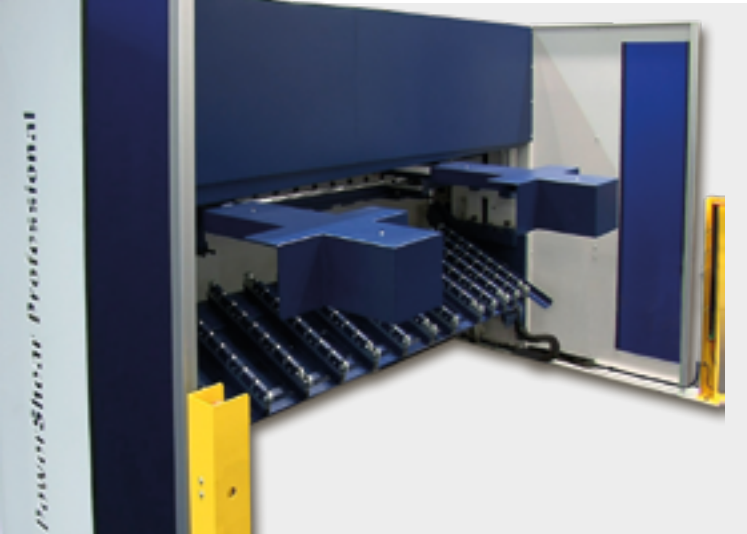
Rückansicht: Motorischer Hinteranschlag und Blechhochhaltevorrichtung sowie Rückraumabsicherung
