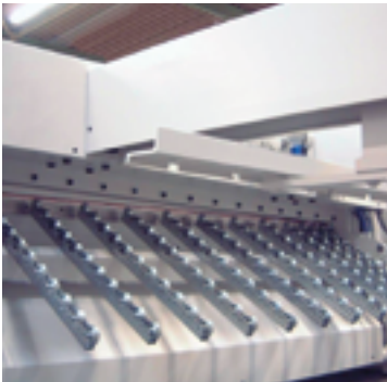
Blechhochhaltevorrichtung pneumatisch gesteuert mit Rollenleisten
