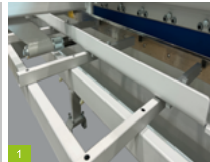
1 Blechochhaltevorrichtung nach vorne in waagerechter Stellung (Variante 1)
