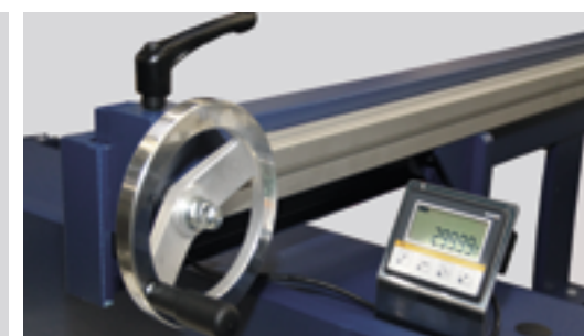
Manueller Hinteranschlag, von vorne verstellbar, mit Digitalanzeige (Standardausstattung)
