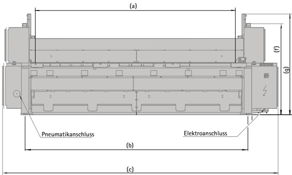
Maße: PDC-NC
