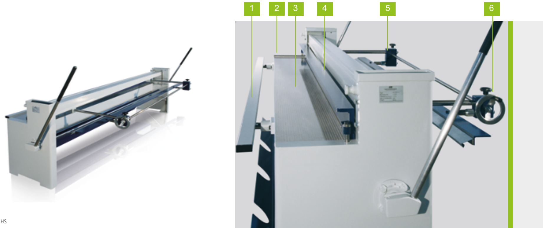
Manueller Hinteranschlag mit Skala und Handradverstellung [6] für parallele und konische Schnitte. Die Einstellung wird an den Winkelführungen [5] durchgeführt.
