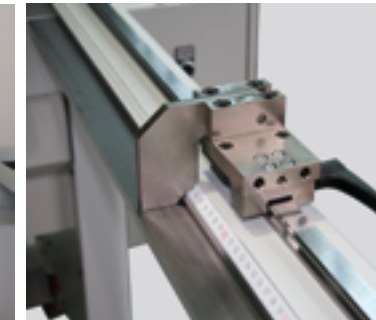
Optional: Verlängerter Winkelanschlag (rechts oder links) mit Maßstab incl. seitlichem Klappanschlag auf Linearführung
