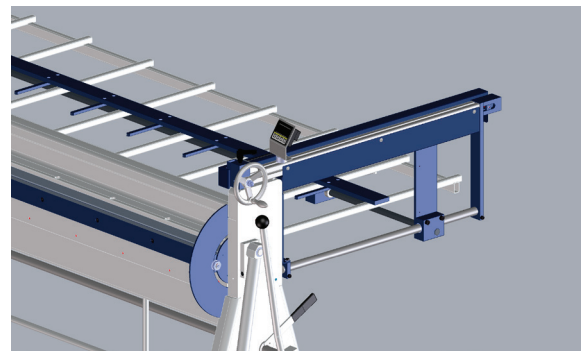
Mit der neuen Option erspart sich der Bediener den Gang um die Maschine, weil er direkt von vorne das Anschlagmaß exakt einstellen kann.
