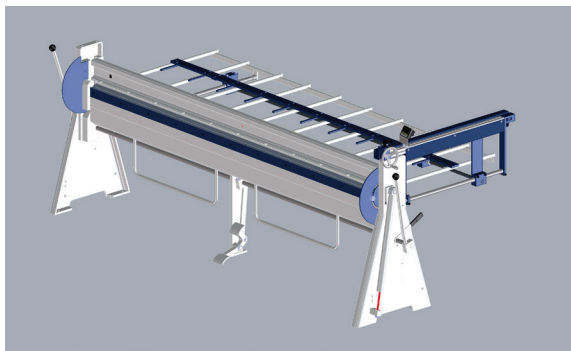
Manueller Hinteranschlag 10 – 750 mm, von vorne verstellbar mit Digitalanzeige incl. Auflagetisch.
