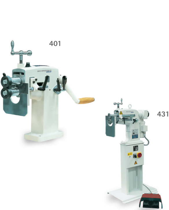
Sicken- und Bördelmaschine 401 mit Handantrieb – geteilter Anschlag und Vornehmwalzen
